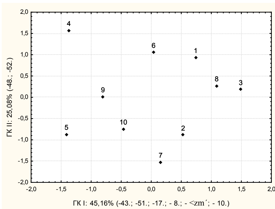
Рис. 1. Взаимное расположение мужских черепов в пространстве двух первых ГК
