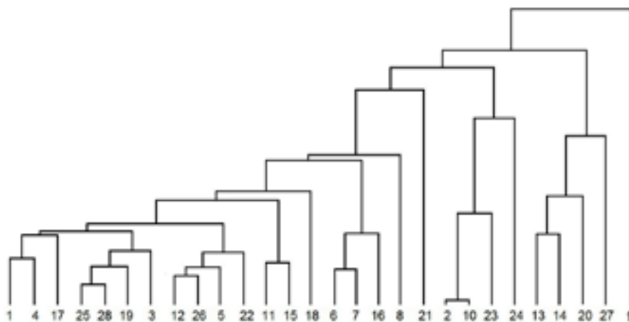
Рис. 19. Компонентный анализ мужских серий эпохи неолита и палеометалла из Средней Азии (ГК I – 1, 45,48 (25,1%); ГК II – 8, 77, SS – (21,8 %); общее 46,9 %).
